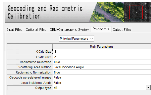
図 26. ジオコーディングダイログの Parameters タブ
